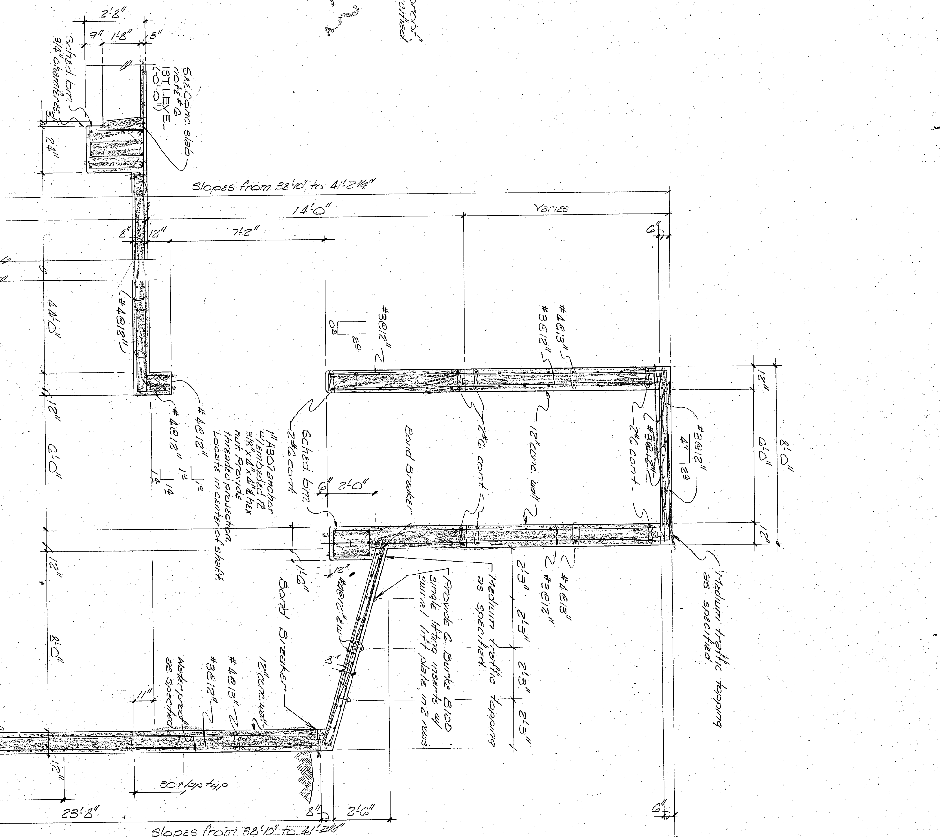
SECTION 2 Scale: 3/8"=1'-0"
