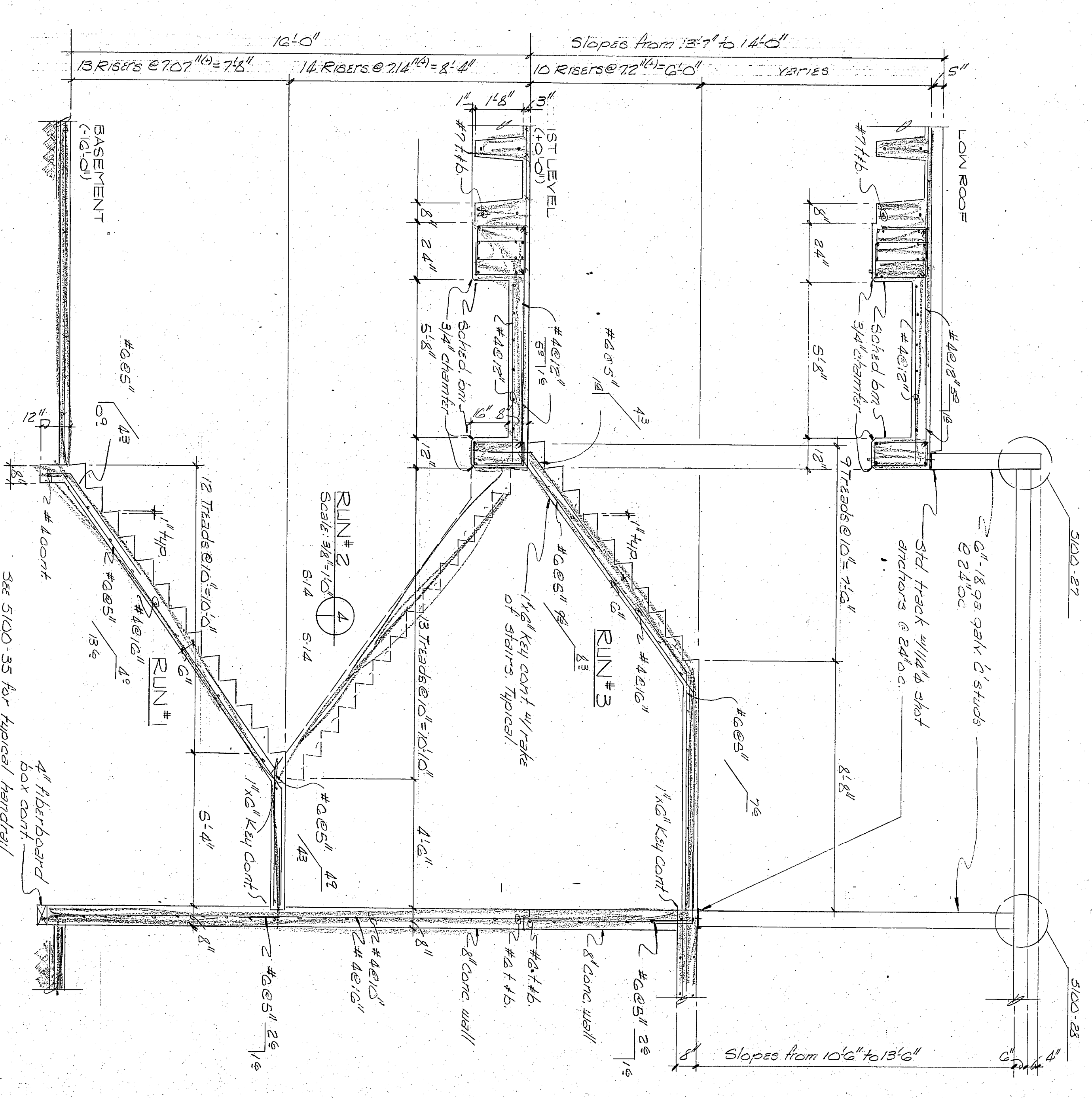
SECTION Scale: 3/8"=1'-0" 5/4
